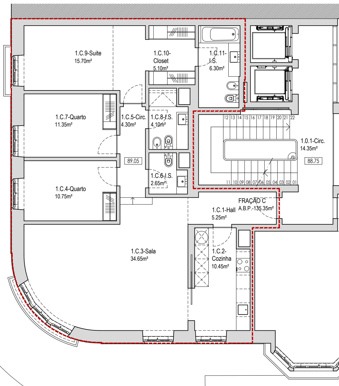
Planta Piso 1 - FRAÇÃO C A. bruta Privativa = 135.35 m 2
