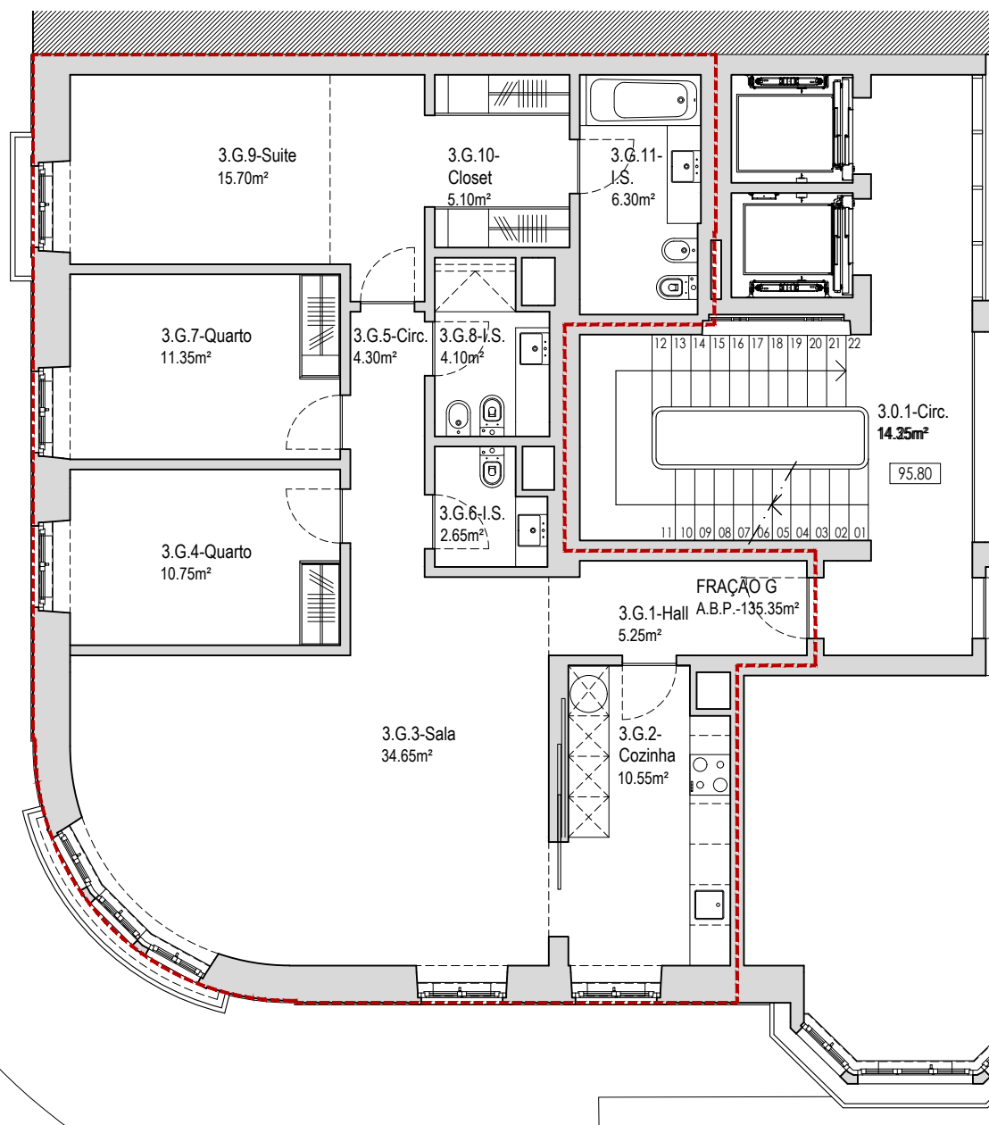
Planta Piso 3 - FRAÇÃO G A. bruta Privativa = 135.35 m 2
